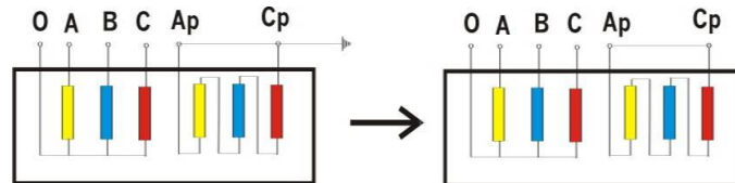
图 3 平衡绕组接线
