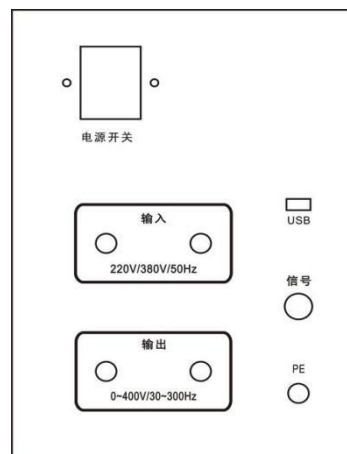
图1-2 侧面接线图
