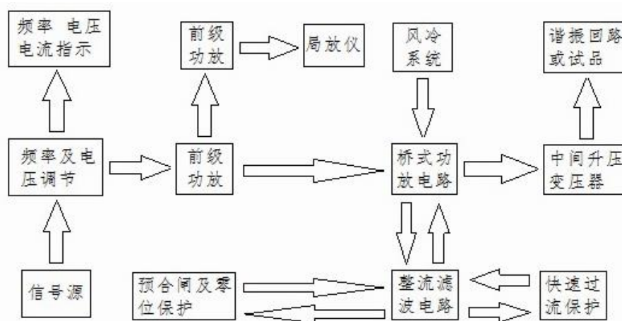
图1 HMCXZW 型变频电源装置工作原理流程图
