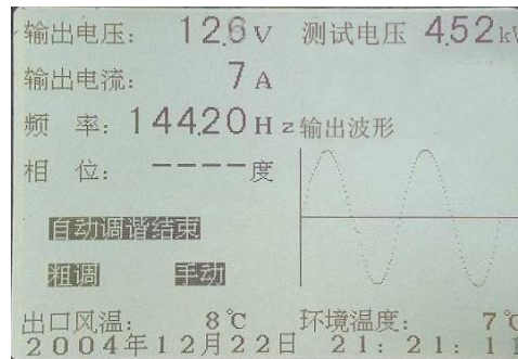
图 26 HMCXZW 变频电源装置自动调谐结束显示
