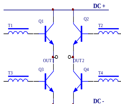
图2 HMCXZW 型变频电源装置桥式放大电路原理图
