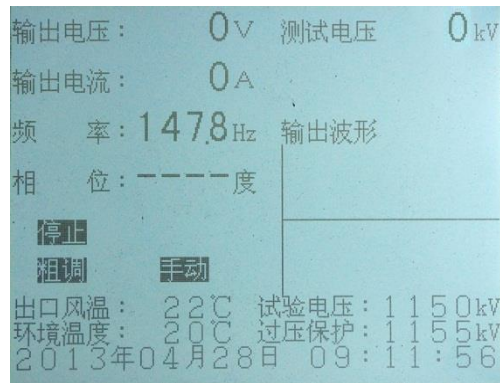
图 18 HMCXZW 型变频电源装置工作界
