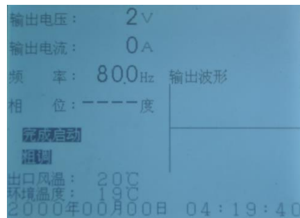
图 22 HMCXZW 变频电源装置启动完成
