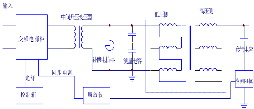
图 31 HMCXZW 型变频电源装置进行局部放电试验接
