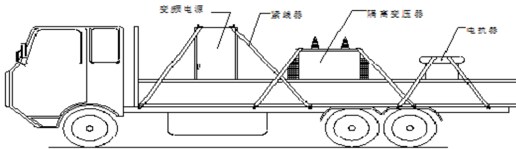
图 36 HMCXZW 型变频电源装置运输示意图
