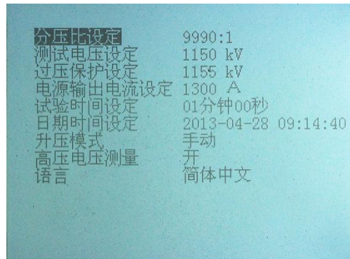
图 19 HMCXZW 变频电源装置菜单
