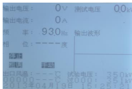
图 37 HMCXZW 变频电源装置调试界面图
